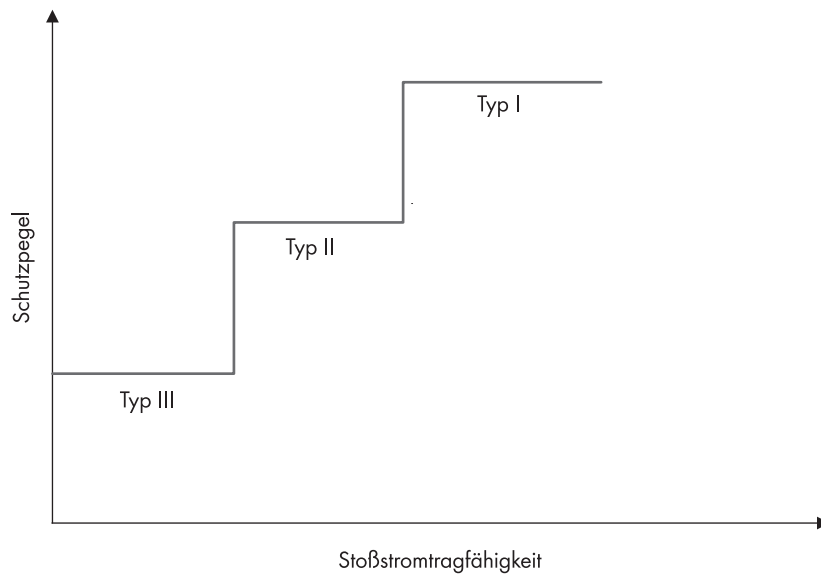
Abb. 2: Schutzpegel von SPD mit unterschiedlicher Stoßstrombelastbarkeit
