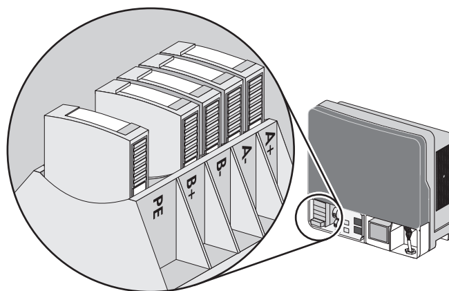
Abb. 7: Installationsort der SPD am Beispiel der Gerätefamilie STP XX000TL-10
