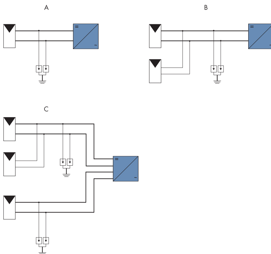
Abb. 3: Ein PV-String an einem Wechselrichter mit einem MPP-Tracker (A), mehrere PV-Strings an einem Wechselrichter mit einem MPP-Tracker (B), mehrere PV-Strings an einem Multi-String-Wechselrichter mit mehreren MPP-Trackern (C)
