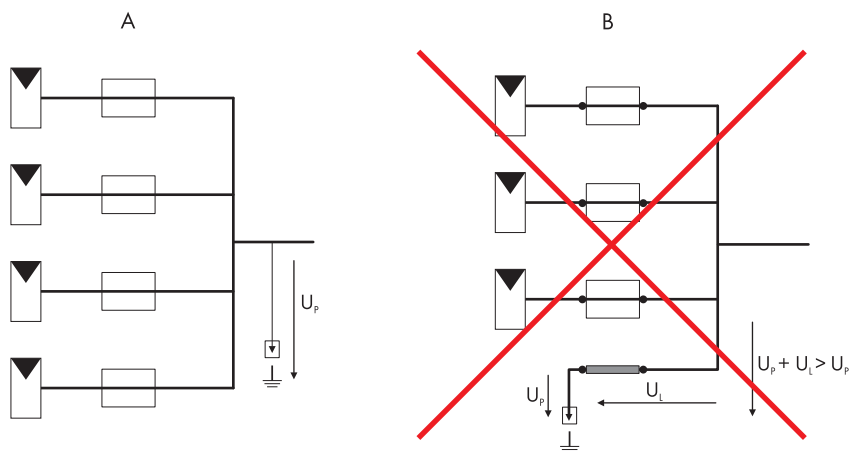
Abb. 6: Den Stringsicherungen nachgeschalteter SPD (A) und SPD an einem Stringeingang, dessen Stringsicherung durch einen Kupferbolzen ersetzt ist (B)
