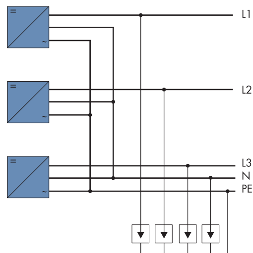
Abb. 4: AC-seitiger Anschluss mehrerer Wechselrichter an ein 3-phasiges Überspannungsschutzgerät
